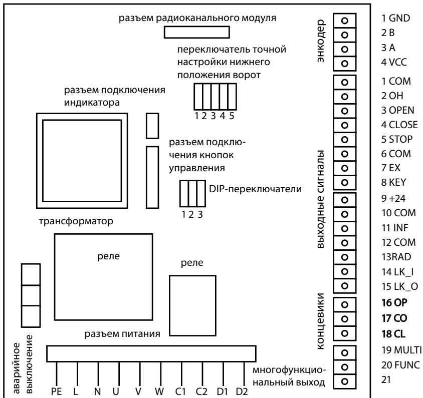
Рис. 11 Расположение элементов на плате GYK-92SY
