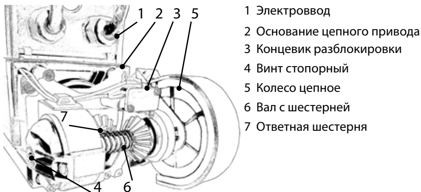
Рис.6 Устройство ручного цепного привода (крышка снята)
