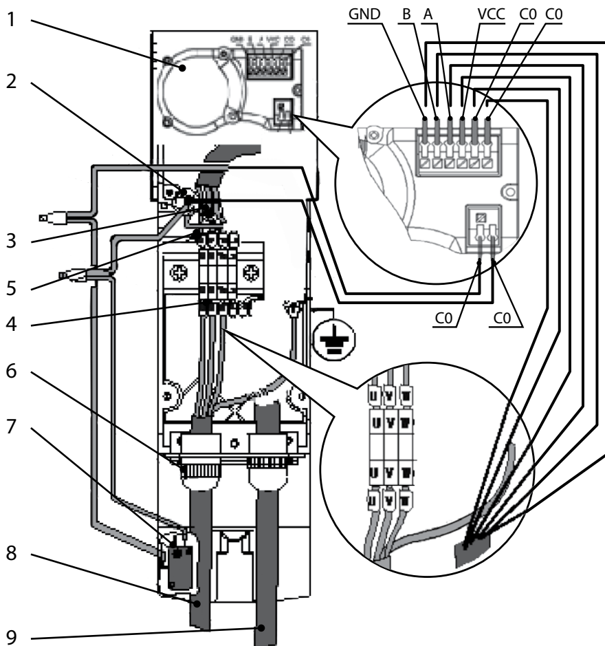
Рис. 8 Схема подключения привода
