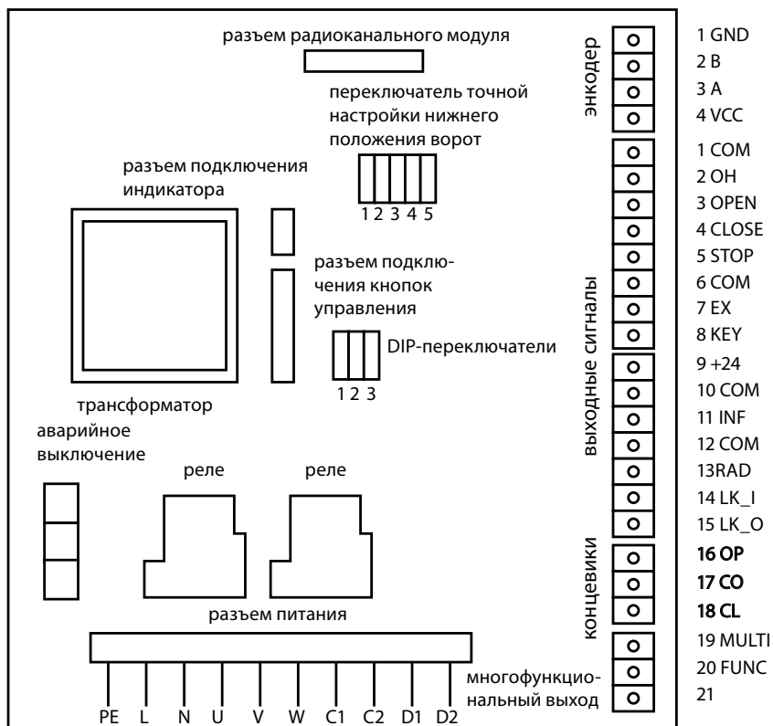
Рис. 10 Расположение элементов на плате ГYК-92Y
